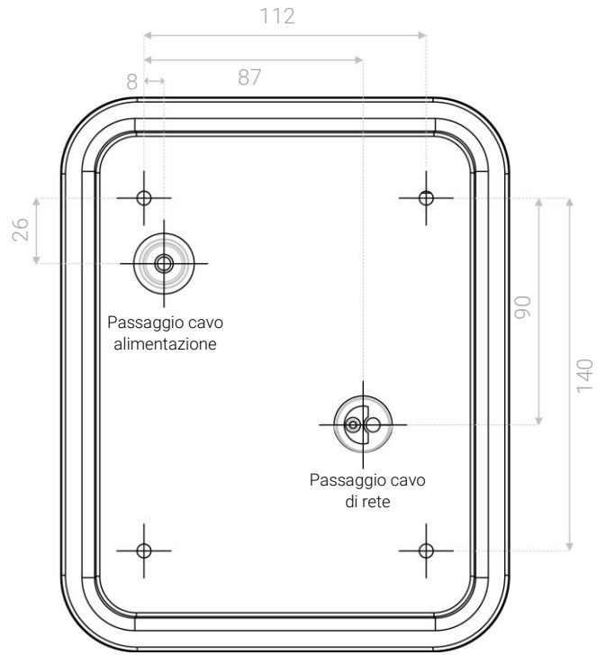
vista posteriore
