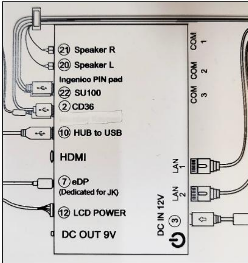
Schema collegamenti CPU
