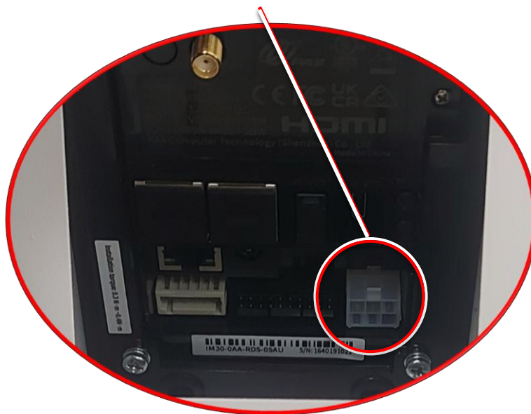
Connettore "POWER" dispositivo di pagamento
