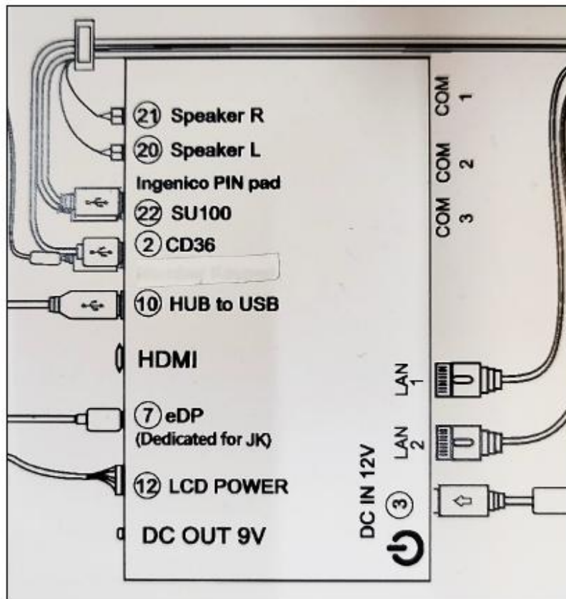
Schema collegamenti CPU
